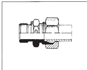
C-GE-R/M zyl. Gerade-Einschraubverschraubungen Male stud couplings Racores rectos
