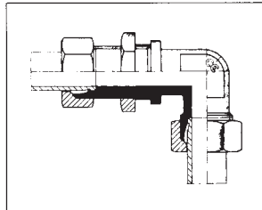
C-WSV Winkel-Schottverschraubungen Bulkhead elbow couplings Uniones en codo pasatabiques
