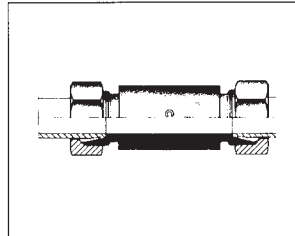
C-ESV Einschweiß-Schottverschraubungen Welding bulkhead couplings Uniones rectas pasatabiques para soldar
