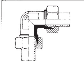
C-W Winkel-Verschraubungen Equal elbow couplings Codos iguales
