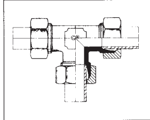
C-T T-Verschraubungen Equal tees Tees iguales
