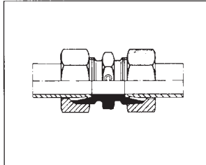
C-G Gerade-Verschraubungen Straight couplings Uniones dobles
