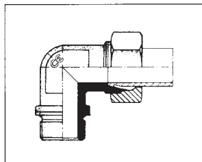
C-WE-R/M zyl. Winkel-Einschraubverschraubungen Male stud elbows Racores en codo
