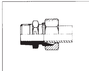
C-GE-R/M keg. Gerade-Einschraubverschraubungen Male stud couplings Racores rectos
