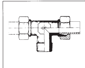
C-TE-R/M keg. T-Einschraubverschraubungen Male stud brunch tees Racores en T, rosca central
