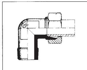
C-WE-R/M keg. Winkel-Einschraubverschraubungen Male stud elbows Racores en codo
