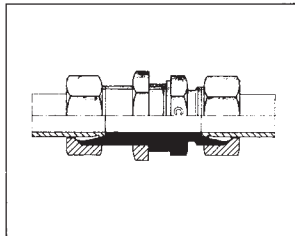
C-SV Gerade-Schottverschraubungen Straight bulkhead couplings Uniones rectas pasatabiques
