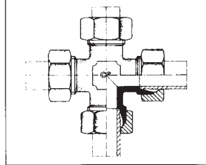
C-K Kreuz-Verschraubungen Equal cross Cruces iguales
