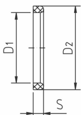
Dichtring DIN 11851 hohe Ausführung sealring
