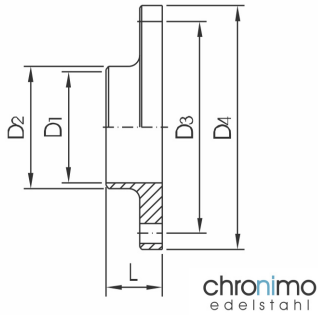
SV-Flansch ohne Nut BV-flange without nut
