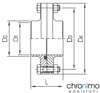
SV-Flanschverbindung BV-flange connection
