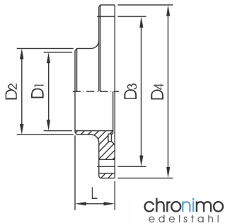
SV-Flansch mit Nut BV-flange with nut
