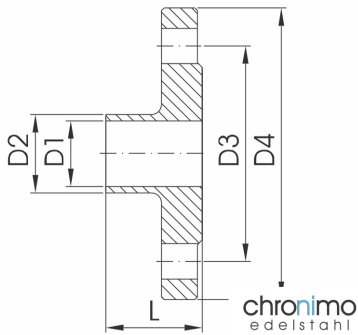
Vorschweißflansch welding neck flange
