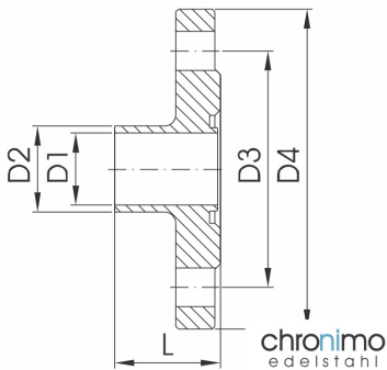
Vorschweißflansch mit Nut welding neck flange with nut
