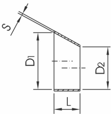
Reduzierstück exzentrisch DIN 11852 reducer-DIN-welding ends excentr.
