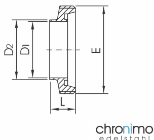
Kegelstutzen DIN 11851 kurz liner (short)
