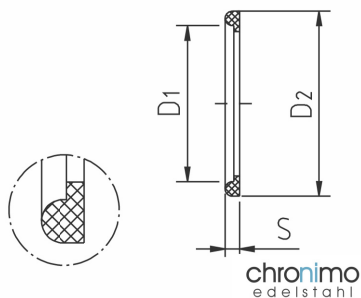
Dichtring DIN 11851 mit Bund sealring
