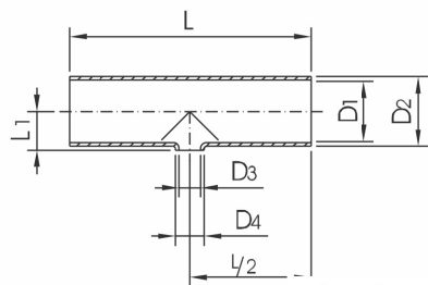
Reduzier T-Stück SSS reducing tee SSS
