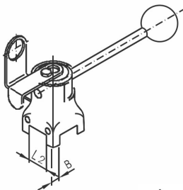
SV-Handgriff für Näherungs-INI (NI) btfl. valve hdl for prox. switch
