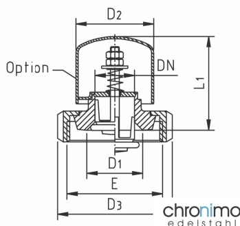
Vakuumventil vacuum valve
