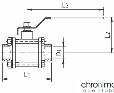
Kugelhahn 3tlg. Gewinde/ Gewinde port ball valve
