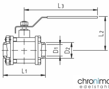
Kugelhahn 3tlg. Schweiß/ Schweiß port ball valve
