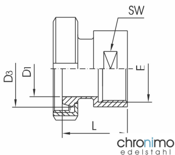
Kegel-Aufschraubstutzen female thread liner
