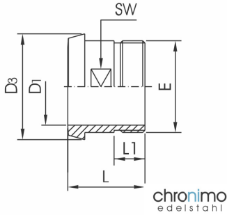
Kegel-Einschraubstutzen male thread liner adapter
