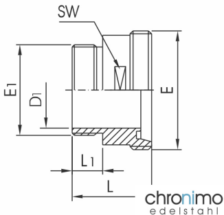
Gewinde-Einschraubstutzen male part adapter
