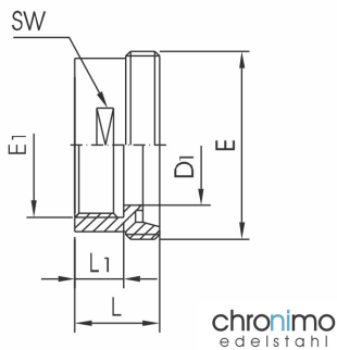
Gewinde-Aufschraubstutzen female part adapter
